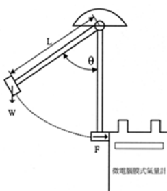
圖 1 衝擊測試
